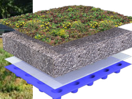
Mix de Sedum Sustrato Geotextil Retenedor de agua
