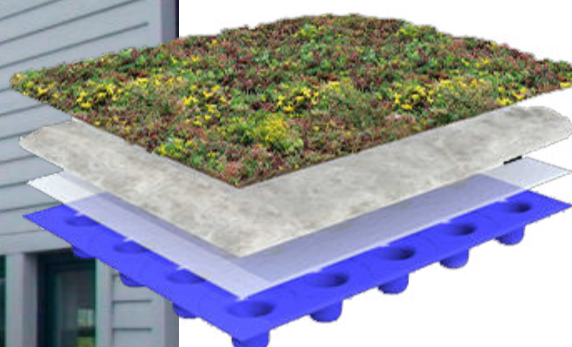
Mix de Sedum Lana de Roca Geotextil
